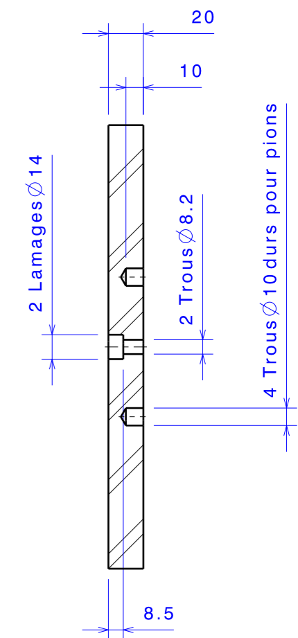
Coupe A-A
